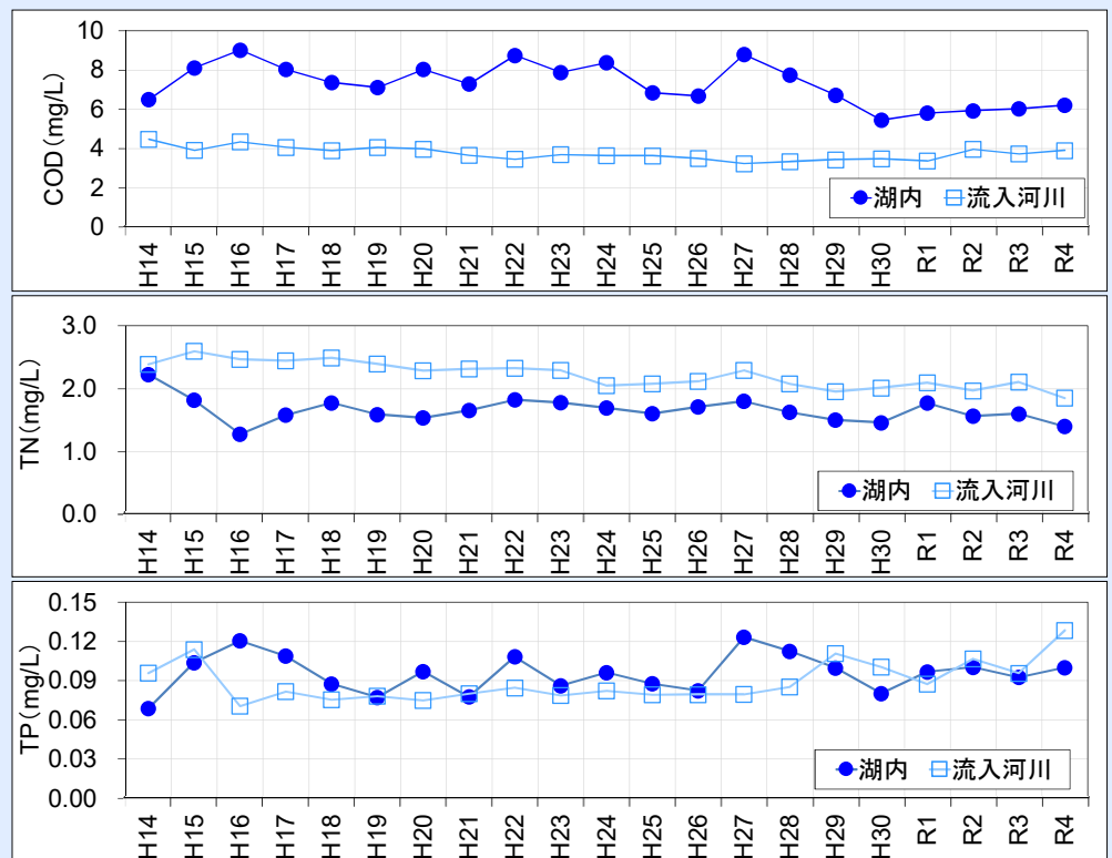
湖内(湖内8地点の平均値)と流入河川(2地点の平均値)におけるCOD(上)、全窒素(中)、全りんの値 ※流入河川は公共用水域の水質測定結果による
